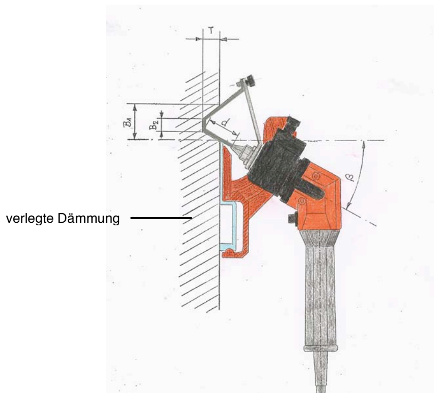
Handschneidegerät TS 11 mit Bossenbügel
